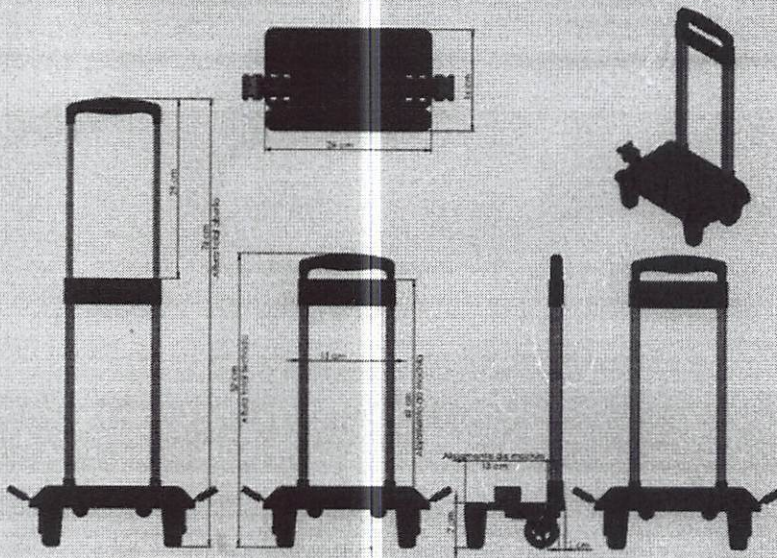
Desenho do Carrinho Removível da Mochila Média
